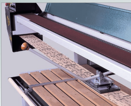
S Brusná odpružená patka • Spring-loaded sanding pad Abgefederter Schleifschuh • Zapata de lija amortiguada Bottine abrasive à ressorts • Поддрессоренная шлифовальная пятка
